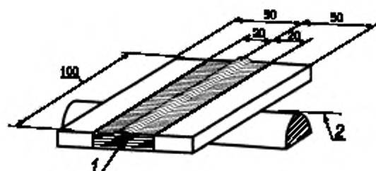
Рисунок Е.1 — Образец для испытаний, сваренный встык
