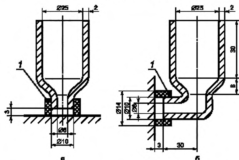
а — сосуд для испытаний горизонтальных поверхностей; б — сосуд для испытаний вертикальных поверхностей;
